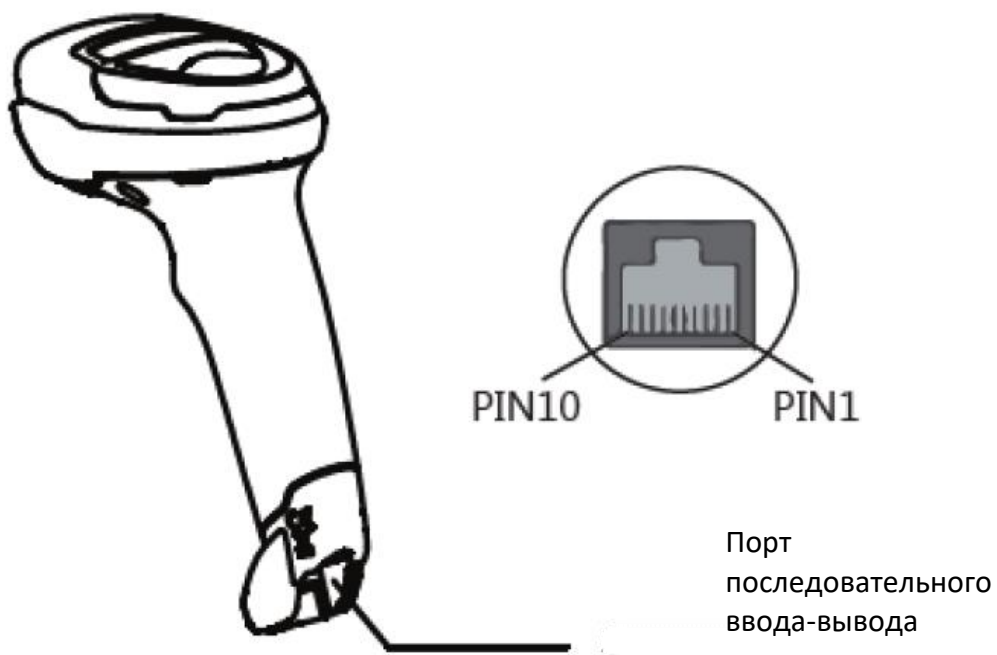
Рисунок 2. Расположение порта последовательного ввода-вывода
