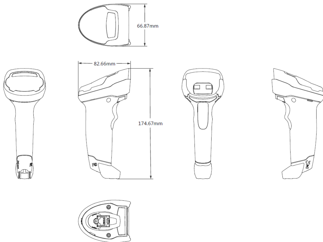
Рисунок 3. Габаритные размеры изделия
