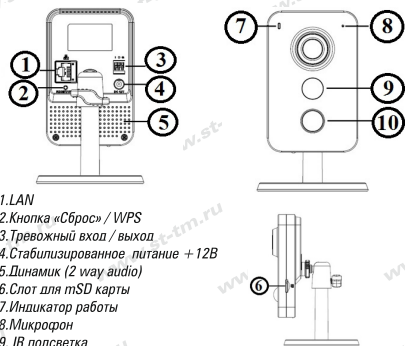
Рис. 1 Схема подключения
