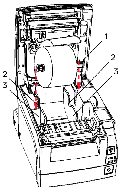
Рисунок 9. Установка ЧЛ с использованием ограничителей
