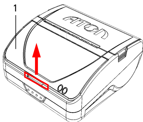
Рисунок 2. Направление приложения усилий при открытии крышки
