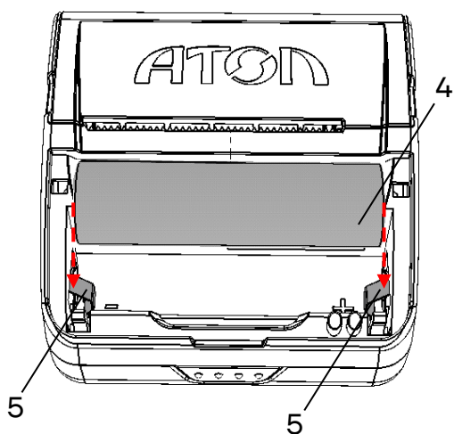
Рисунок 5. Установка аккумулятора
