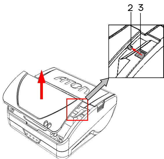
Рисунок 4. Снятие крышки
