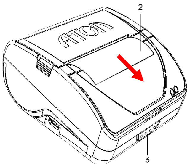
Рисунок 9. Установка ЧЛ в лоток
