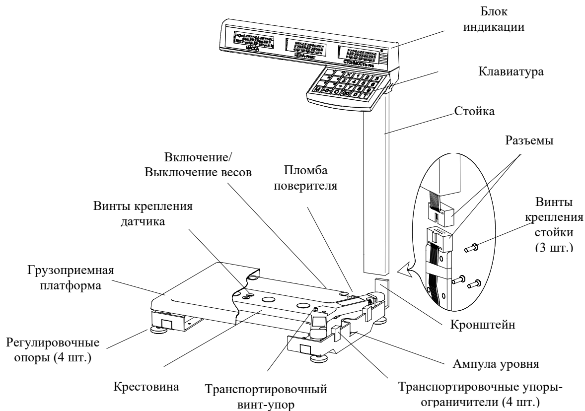
Рисунок 1 – Конструкция весов МК_TV21
