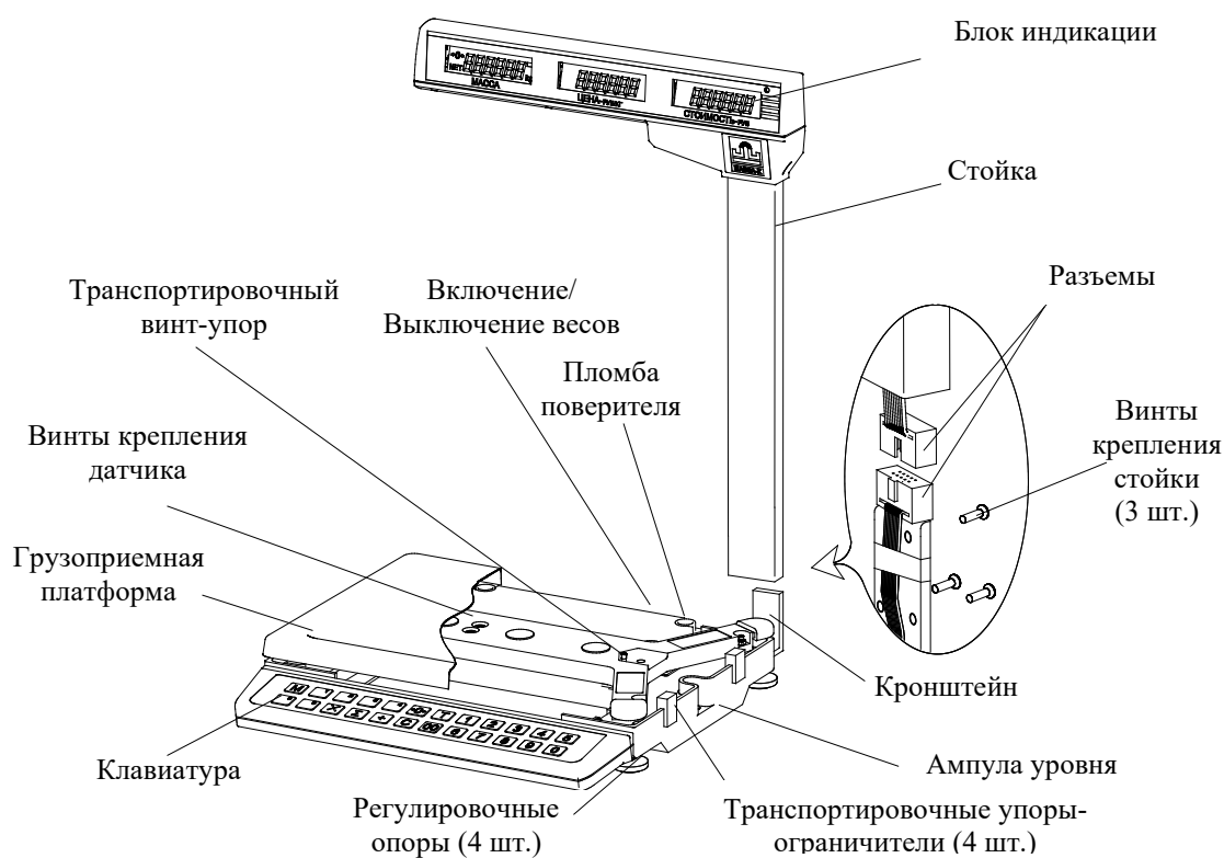
Рисунок 2 – Конструкция весов МК_TN21
