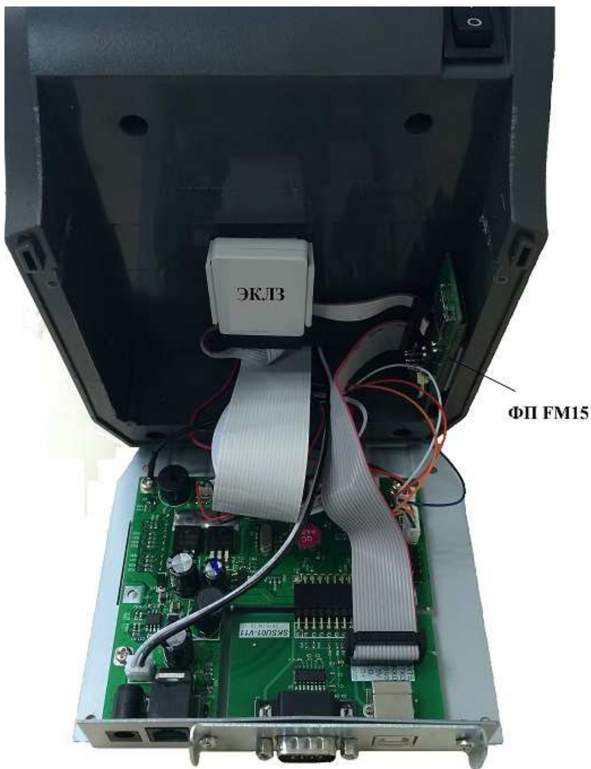
Рис.1 Фото соединения ФП и ЭКЛЗ с системной платой ПТК.
